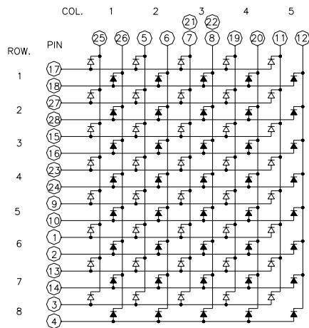
B. LTP-2558AA
