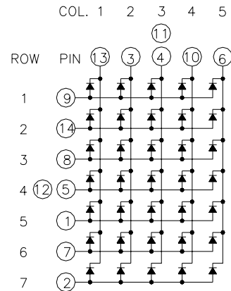
B. LTP-2157A
