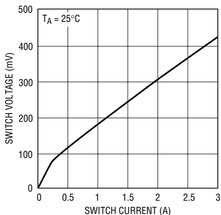
SW1 V_{CESAT}
