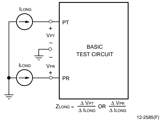
Figure 10. Longitudinal Impedance
