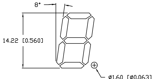
DIGIT DETAIL
