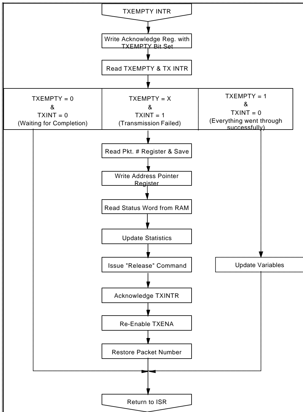
FIGURE 16 – TXEMPTY INTR
