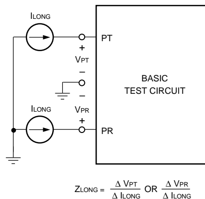
Figure 9. Longitudinal Impedance
