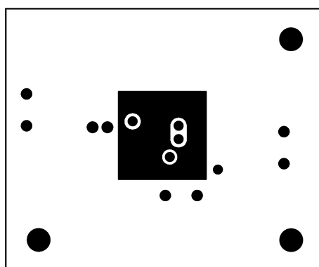
Inner GND Layer
