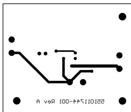
Bottom Layer
