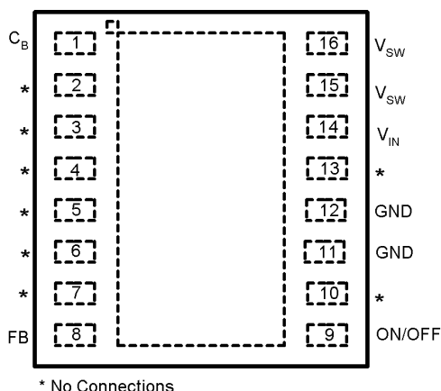
LLP Package
