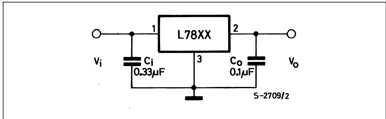
Figure 1 : DC Parameter
