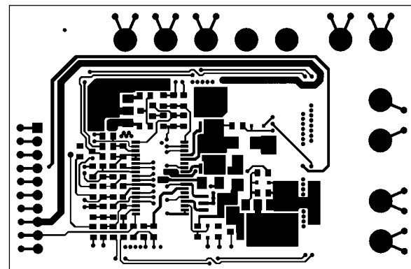
Copper Layer 4
