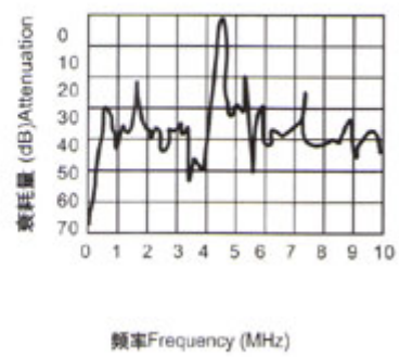
LT4.5MB杂波特性曲线 (0-10MHz) LT4.5MB Spurious Characteristics
