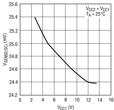
V_{\text{SENSE(SC)}} vs V_{CC1}
