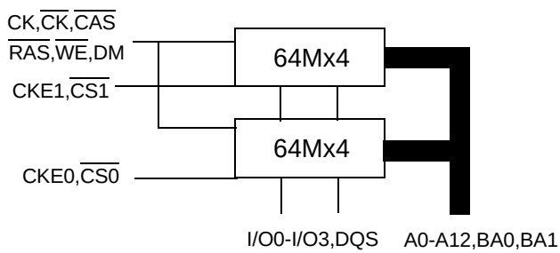
st.128Mb x 4
