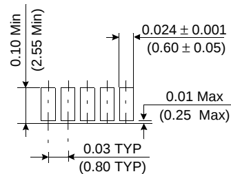
Detail Y
