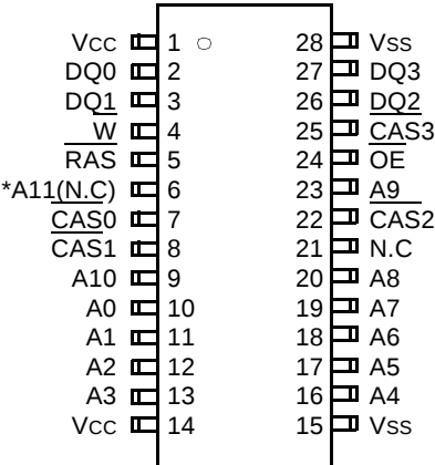
• K4Q17(6)0411C-F
