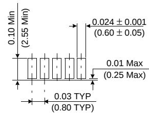
Detail Y
