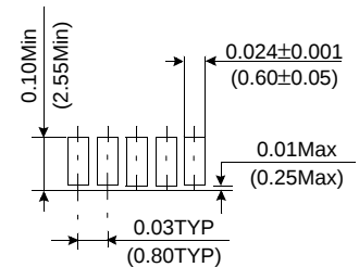
Detail Y
