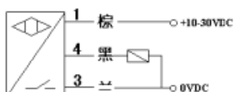
图2：PNP常开或常闭三线输出
