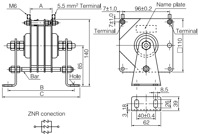
ERZA80JK□□□B
