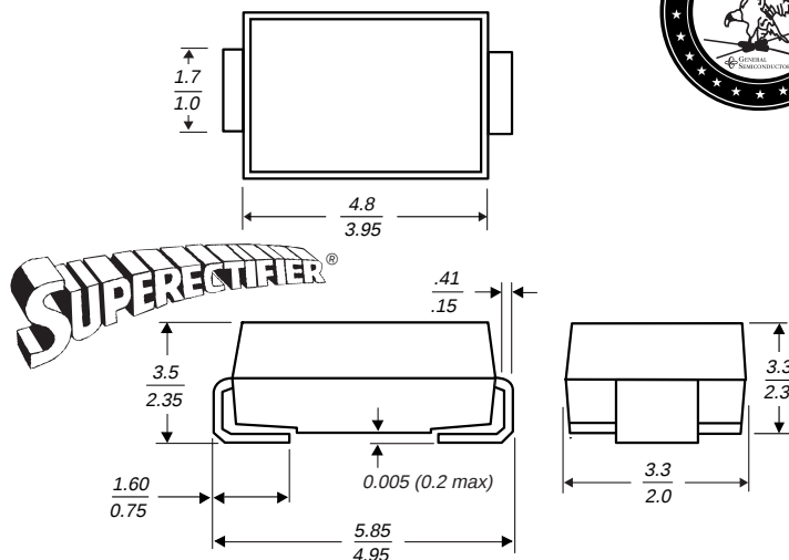
DO-214BA (UEG2)
