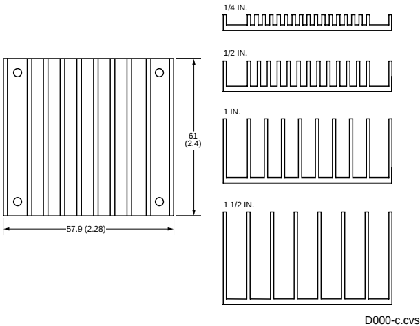
Figure 23. Longitudinal Heat Sink
