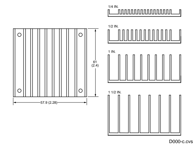
Figure 32. Longitudinal Heat Sink
