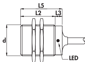
G-1形外壳尺寸
