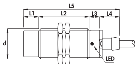
D-2 形外壳尺寸
