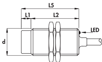
H 形外壳尺寸
