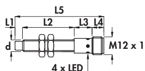
I-11形外壳尺寸
