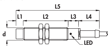
D形外壳尺寸
