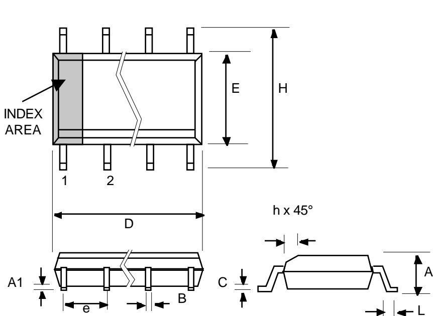
8 pin SOIC
