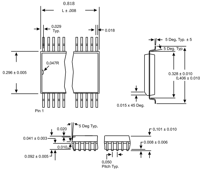
SOIC Package
