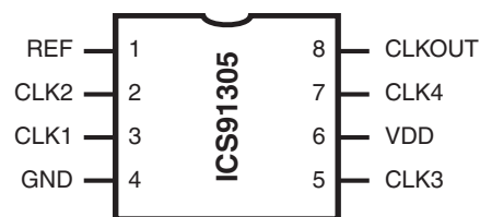
8 pin SOIC
