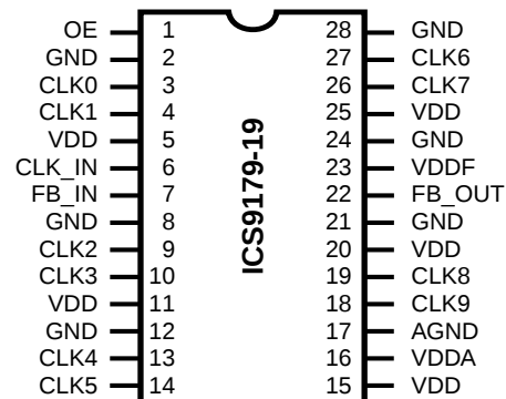
28 Pin SSOP
