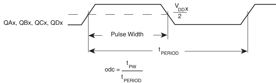
FIGURE 7 - odc & t_{PERIOD}
