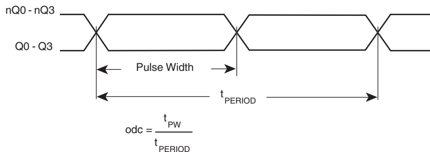
FIGURE 8 - odc & t_{PERIOD}
