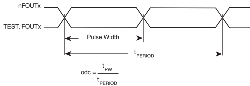
FIGURE 5 - odc & t_{PERIOD}
