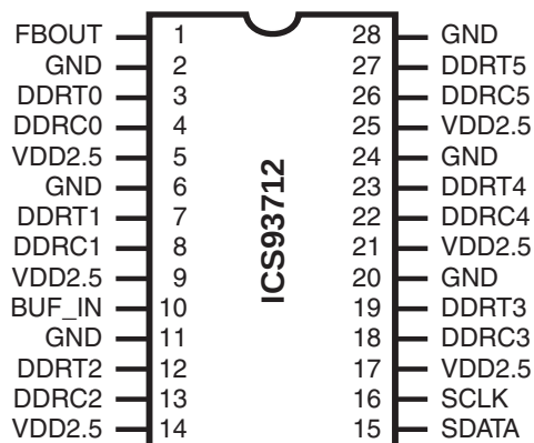
28-Pin SSOP
