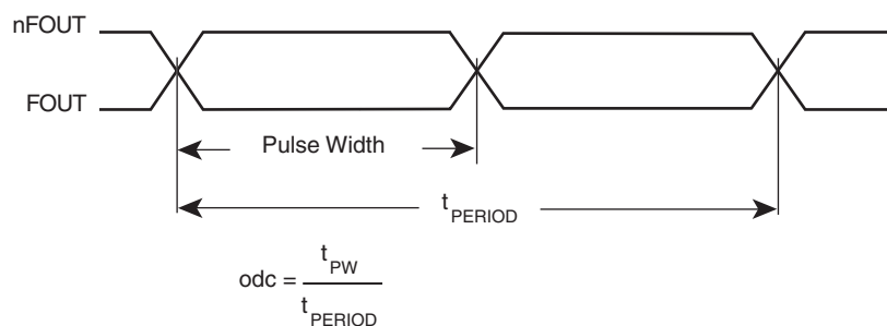
FIGURE 4 - odc & t_{PERIOD}
