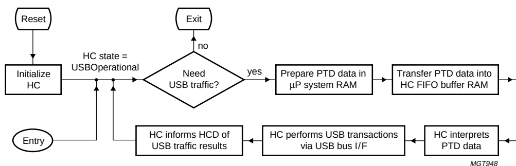
Fig 15. ISP1160 HC USB transaction loop.
