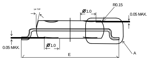
SECTION V-V
