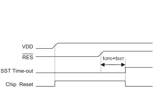
复位时序图
