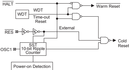
复位框图
