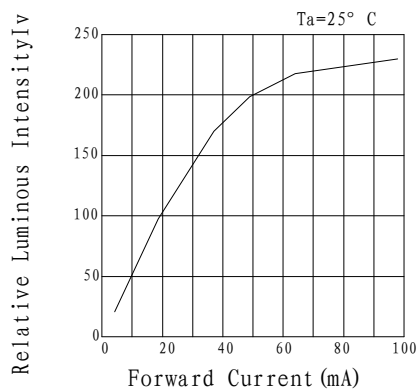
RELATIVE LUMINOUS INTENSITY VS. FORWARD CURRENT 相对光强--正向电流
