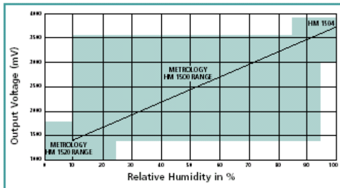
HM1500 模拟电压输出曲线 (Vs=5V)
