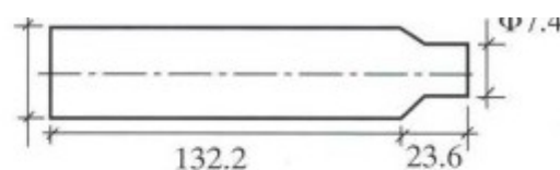
HTP633(S)投入头尺寸
