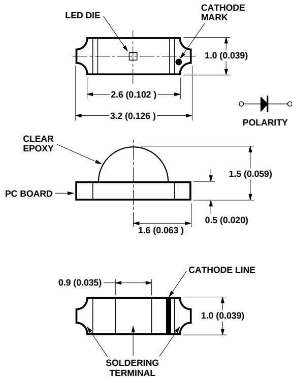
HSMB-C110
