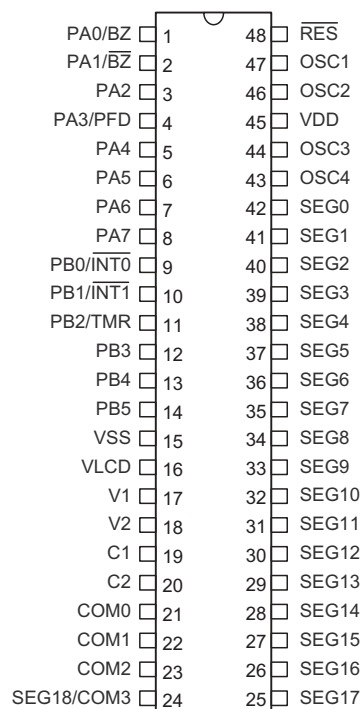
HT49R30A-1 – 48 SSOP-A
