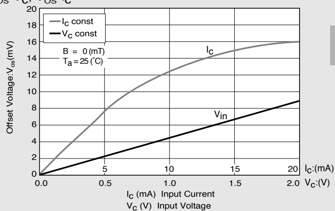
V_{OS} - V_C , V_{OS} - I_C
