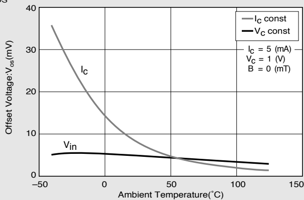
V_{OS} -T
