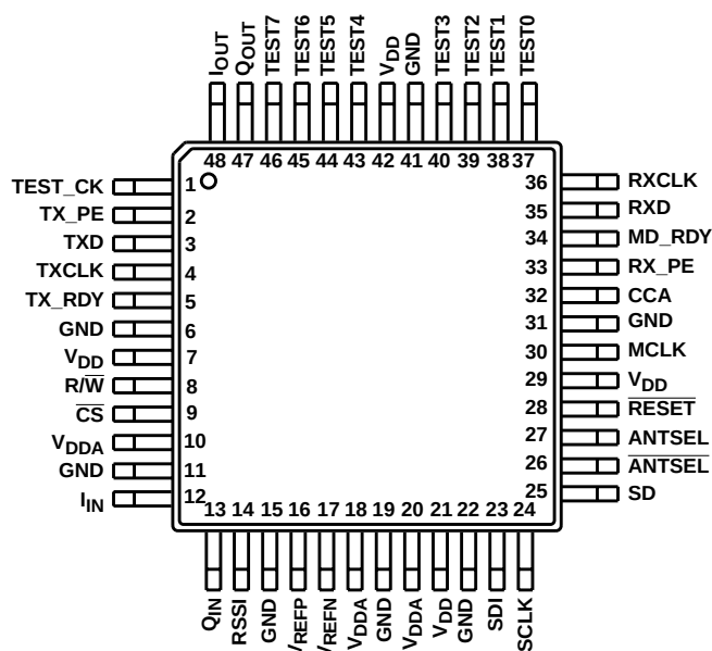
HFA3860B (TQFP)
