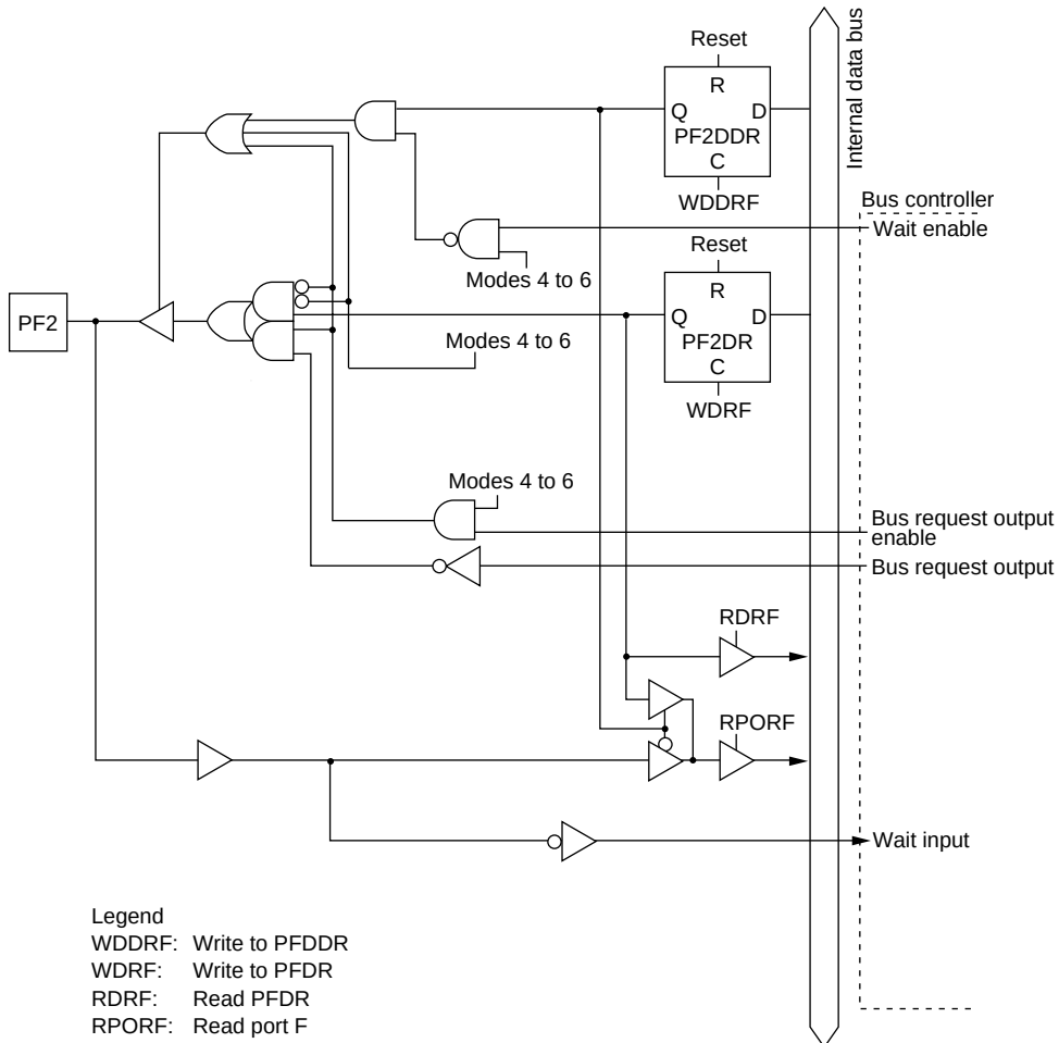
Figure C-9 (d) Port F Block Diagram (Pin PF2)
