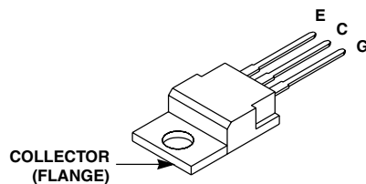
JEDEC TO-220AB
