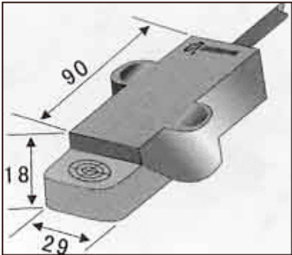
GH1电感式接近开关 ( )
