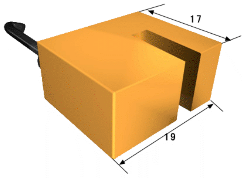
GH1电感式接近开关 ( )
