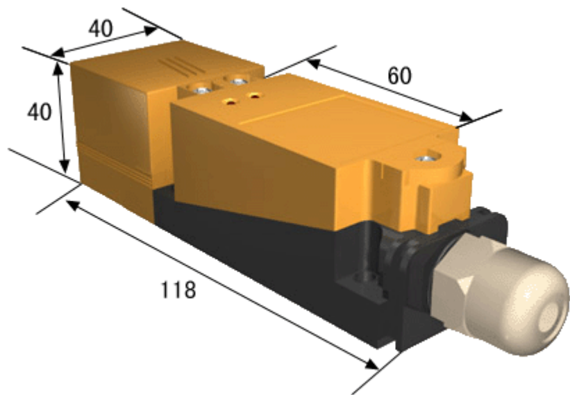
GH1电感式接近开关 ( )
